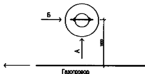
План установки опознавательного столбика
