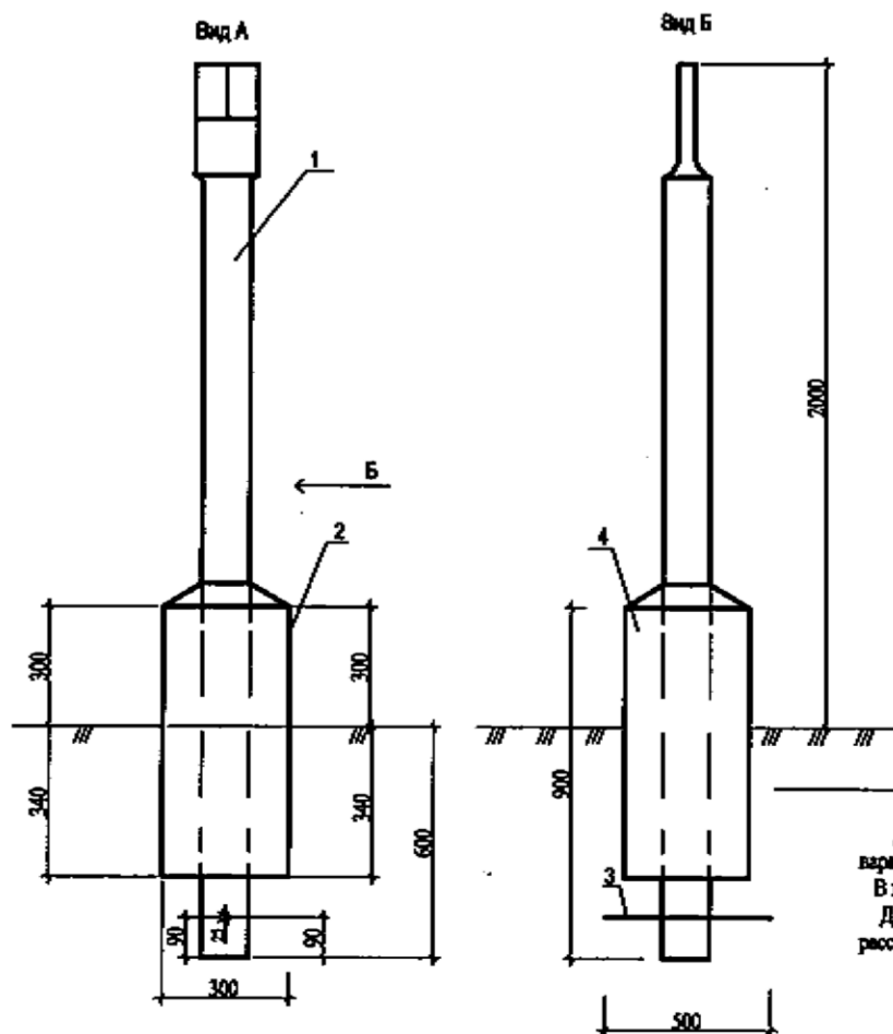
План установки опознавательного столбика
